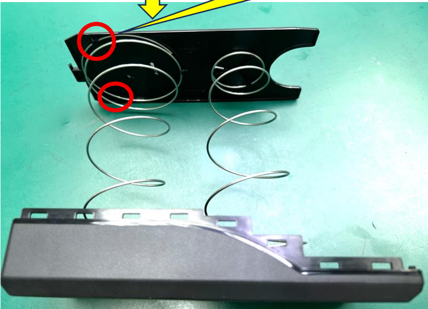
图一，将 PA3580-3 和 PA3580-4 装配在一起，注意装配方向，将弹簧大口位装入卡扣，确保弹簧开口处 2 个扣完全扣入。
