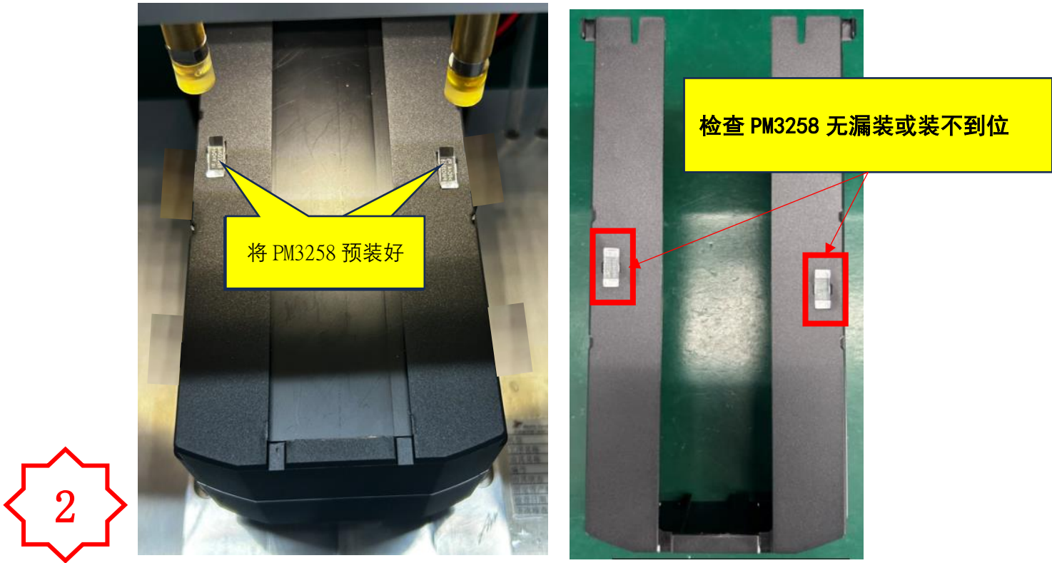
图二，将 PM3088 先放入治具，在将两个 PM3258 预装好，再进行压合， 压合到位后取出检查物料无漏装或压合不到位。
