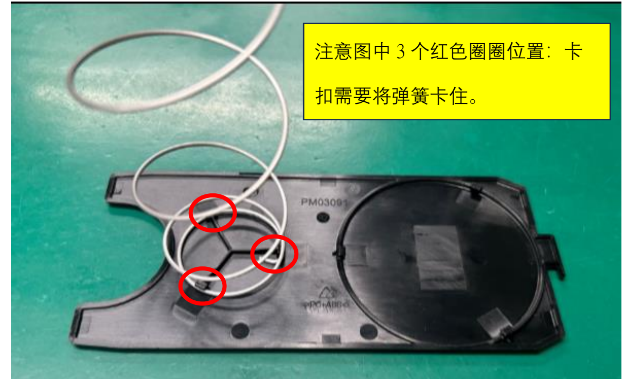
图一，将 SP2422 弹簧小口位装配在 PM3091 对应的位置，注意卡扣要将弹簧卡到位。
